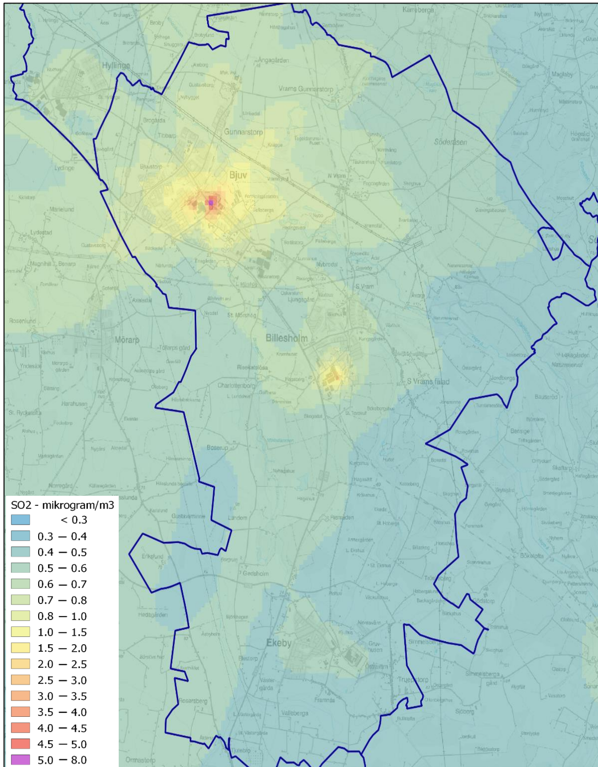
Figur 27. Beräknade årsmedelvärden av svaveldioxid (SO 2 ) inom kommunen (µg/m 3 ).
