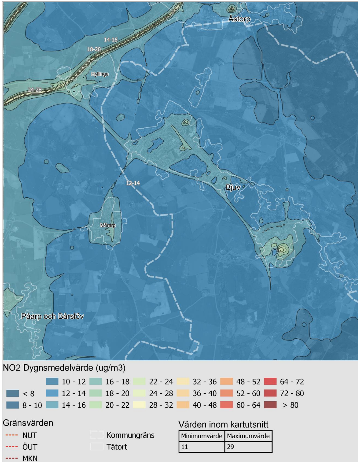
Figur 8. Beräknade dygnsmedelvärderna av kvävedioxid i tätorten ( \mu\text{g}/\text{m}^3 ).
